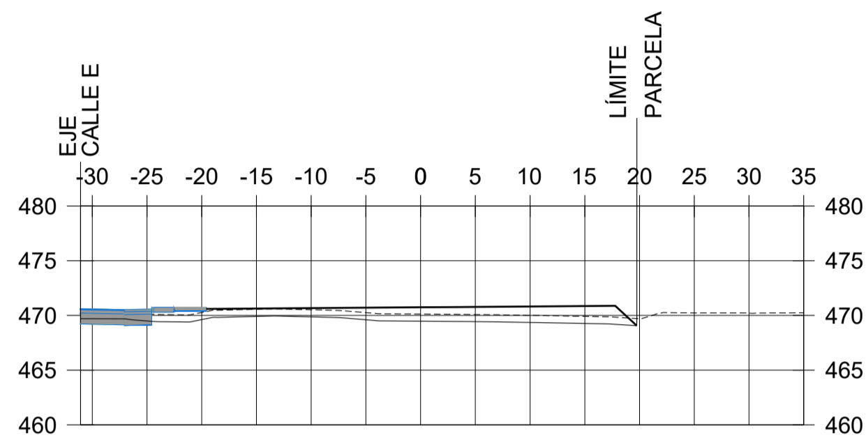
P.K.=0+180
