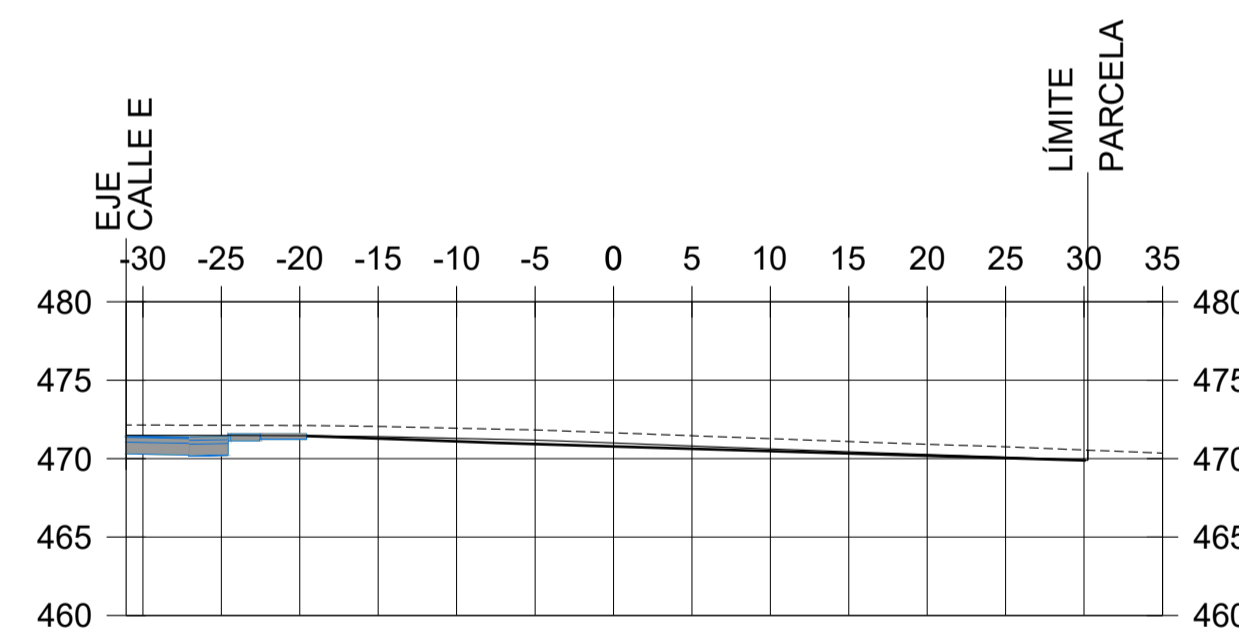
P.K.=0+060
