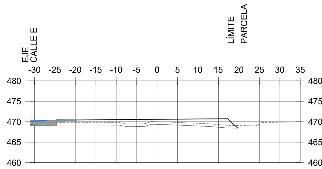
P.K.=0+200
