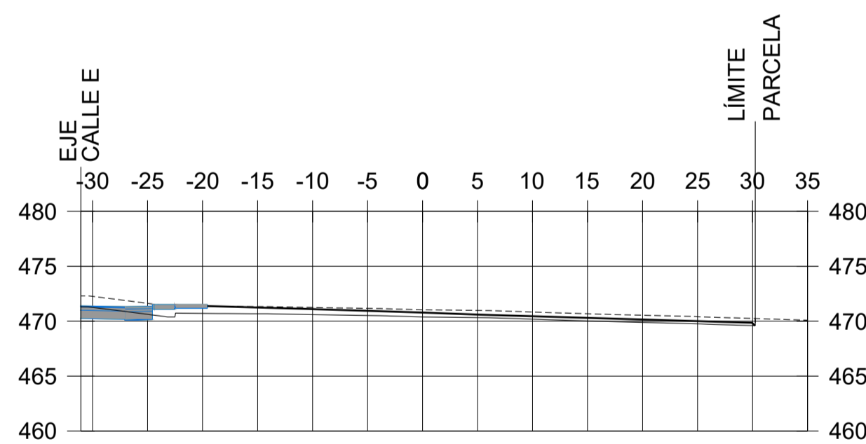
P.K.=0+040
