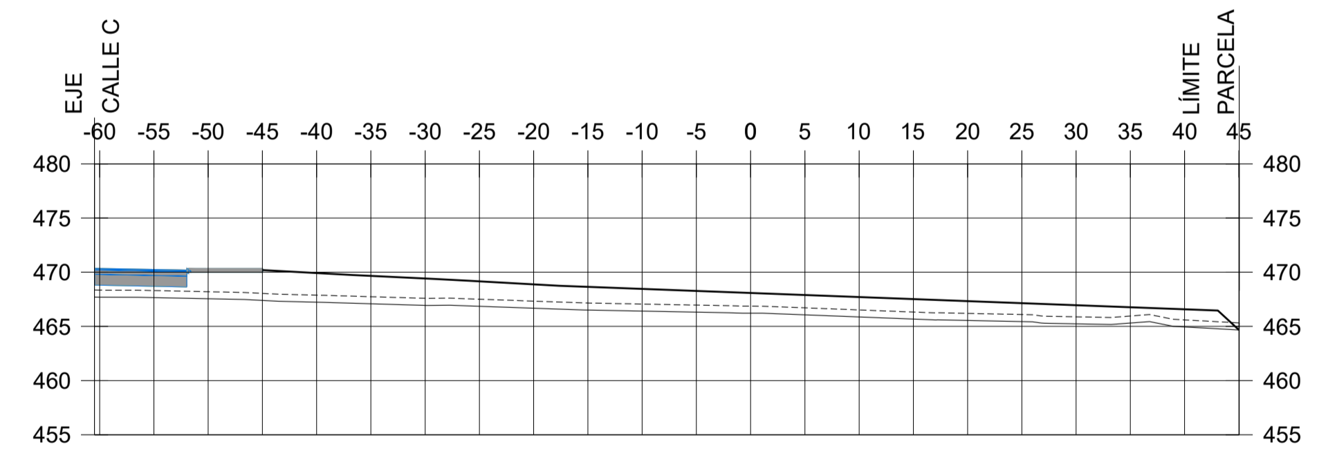
P.K.=0+060
