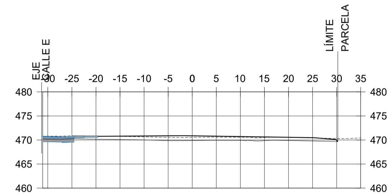
P.K.=0+160
