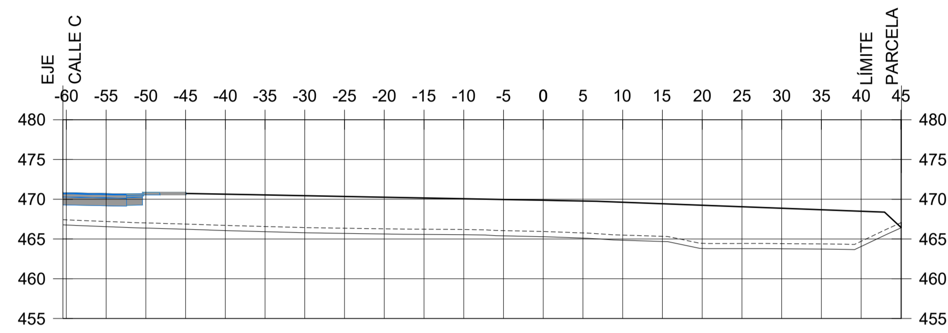
P.K.=0+140
