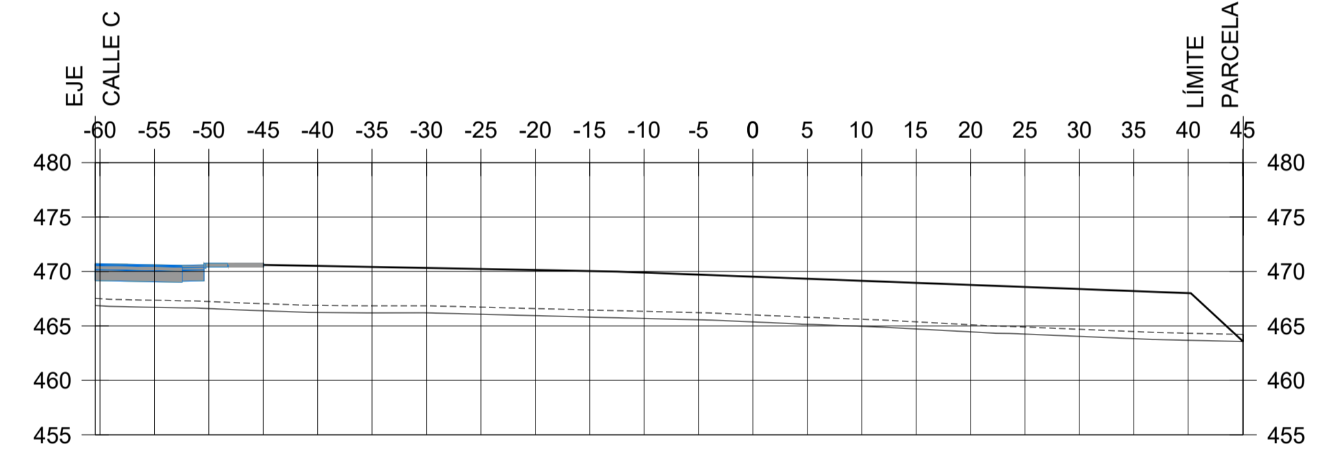
P.K.=0+120
