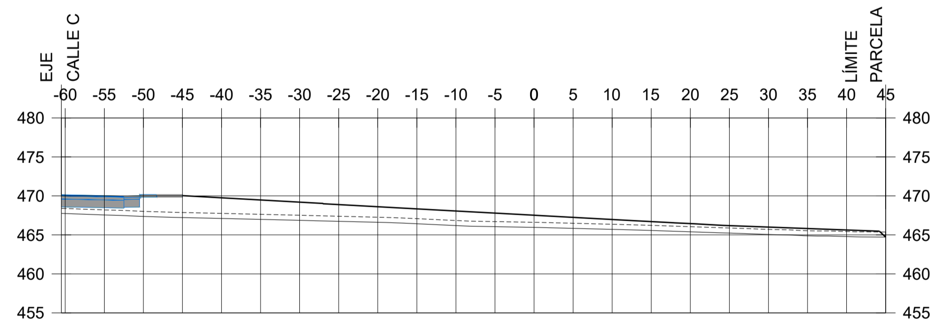
P.K.=0+020
