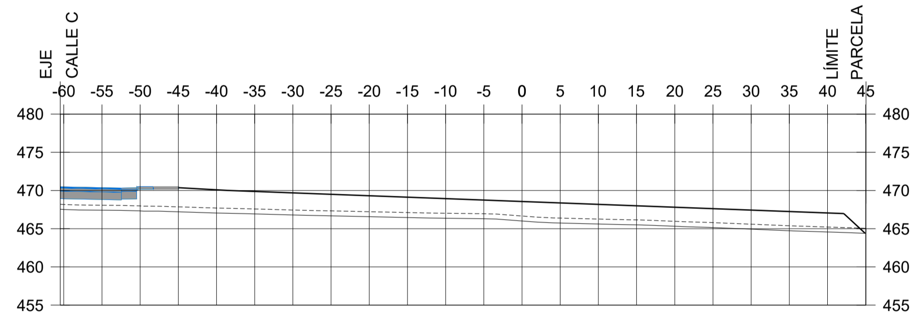
P.K.=0+080
