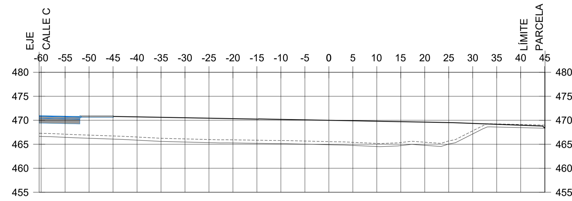
P.K.=0+160
