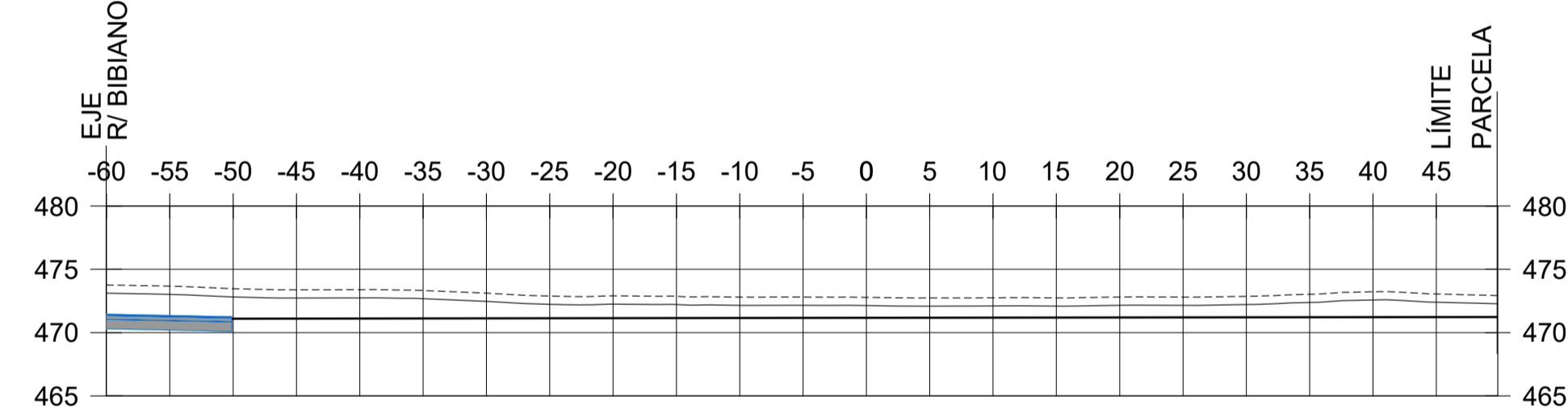
P.K.=0+100
