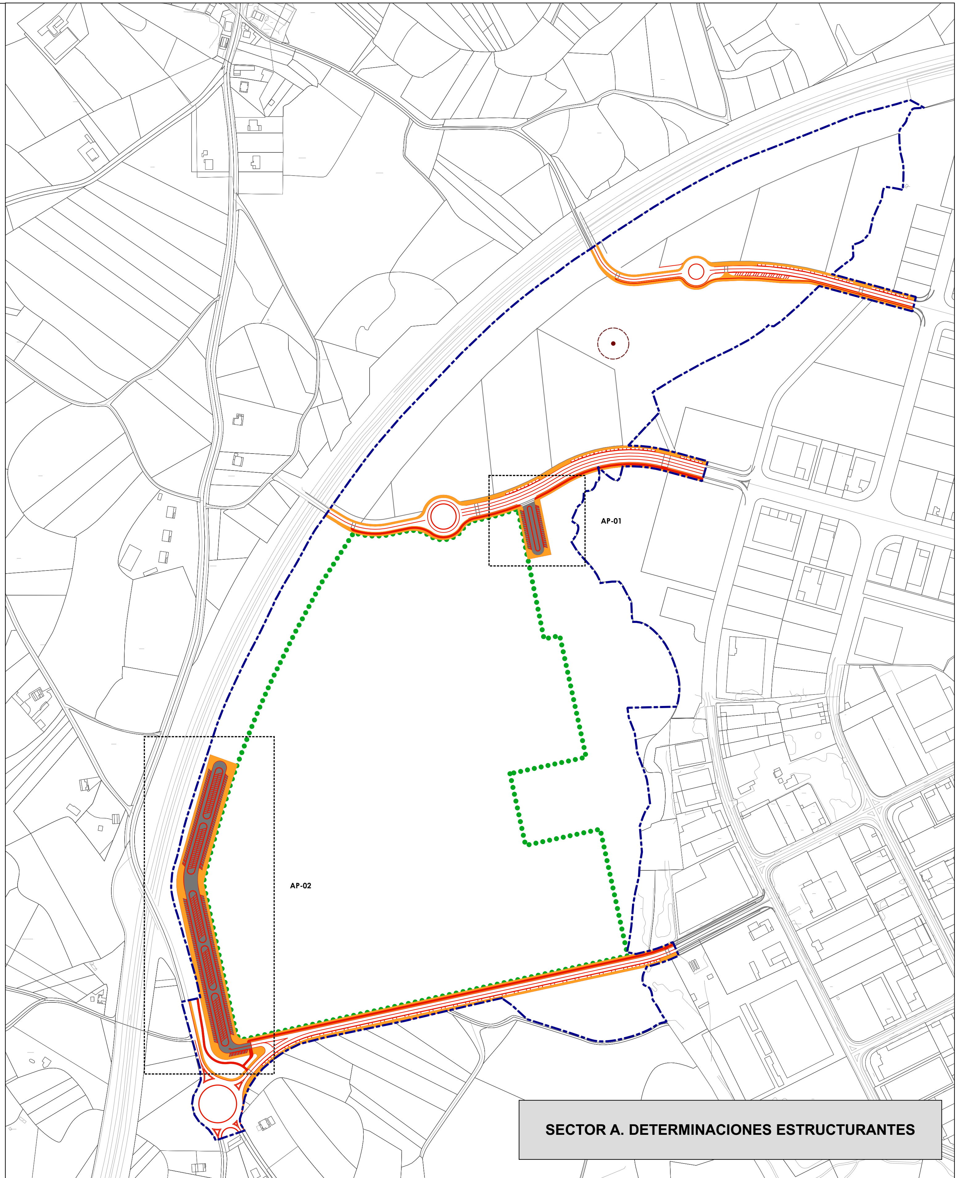
AP-01 ESCALA 1/500
