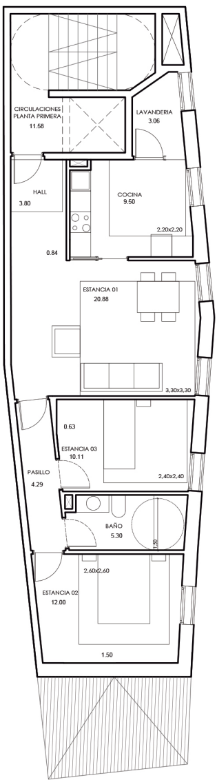
Esc. 1/150 PLANTA TÍPICA EDIFICIO C
