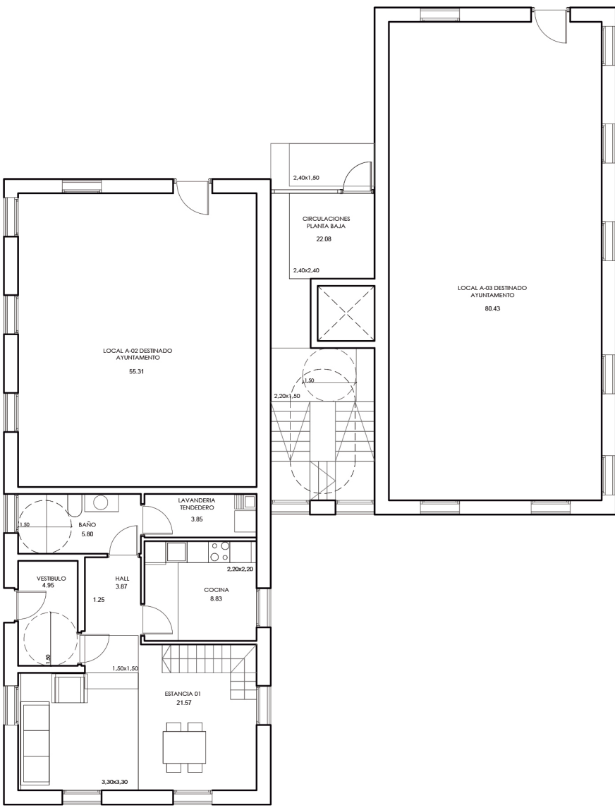
Esc. 1/150 PLANTA BAJA EDIFICIO AB, COTA 0.00
