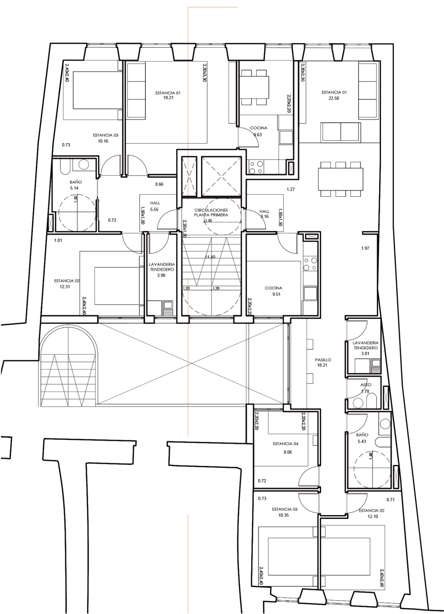
Esc. 1/150 PLANTA MIÑO
