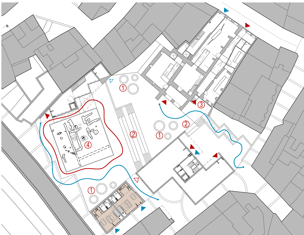
CIRCULACIONES - ACCESOS RELACIÓN CON EL ENTORNO E: 1/600 ■ RECORRIDOS ACCESIBLES ■ RECORRIDO ACCESIBLE VISTAS RESTOS ARQUEOLÓGICOS ■ ACCESOS A EDIFICACIÓN USO TERCIARIO ■ ACCESOS A EDIFICACIÓN USO RESIDENCIAL ■ ÁREAS DE ESTANCIA A LA SOMBRA, BANCOS Y JARDINERAS ■ ÁREAS DE ESTANCIA AL SOL, GRABAS ■ ÁREAS DE USO VINCULADO A PAZO DE DOÑA URRACA ■ RESTOS ARQUEOLÓGICOS VISITALES EN SU NIVEL Y VISIBLES DESDE EL NIVEL DE CALLEJÓN MURALLA
