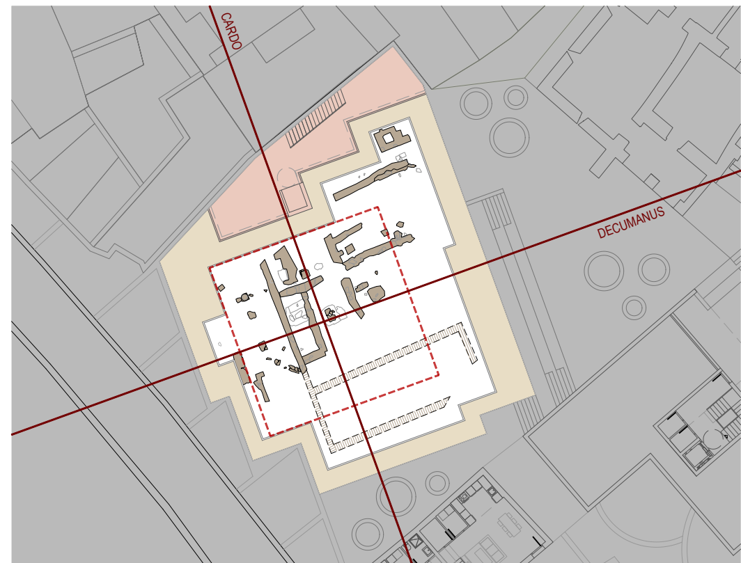
RESTOS ARQUEOLÓGICOS E: 1/400 ■ RESTOS ARQUEOLÓGICOS ANTIGUA VILLA ROMANA ■ TRAZAS PREVISIBLES RESTOS ARQUEOLÓGICOS ■ DIRECCIONES DEL CARDO MAXIMO Y DECUMANUS MÁXIMO DE LA ANTIGUA LUCUS AUGUSTI ■ CENTRO DE INTERPRETACIÓN DE LOS RESTOS ARQUEOLÓGICOS ■ RECORRIDO PERIMETRAL CUBIERTO - VISITA A LOS RESTOS ARQUEOLÓGICOS ■ PROYECCIÓN DE HUECO EN URBANIZACIÓN PARA VISTA DE LOS RESTOS DESDE EL NIVEL SUPERIOR
